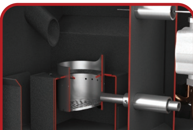
2 Braciore CSS by Laminox. Accensione rapida con candelina ceramica.
